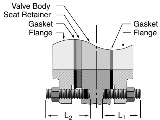
Studs & Hex Nuts
