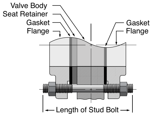
Stud Bolt & 2 Hex Nuts
